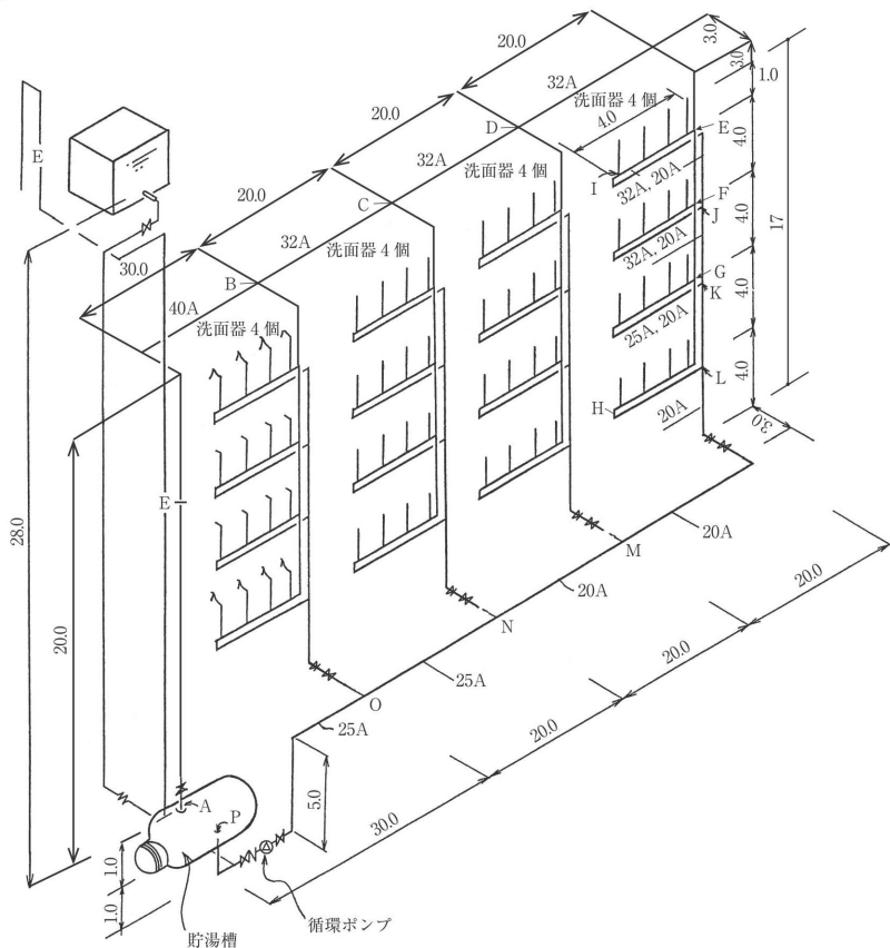
図 5.10 給湯配管系統図
